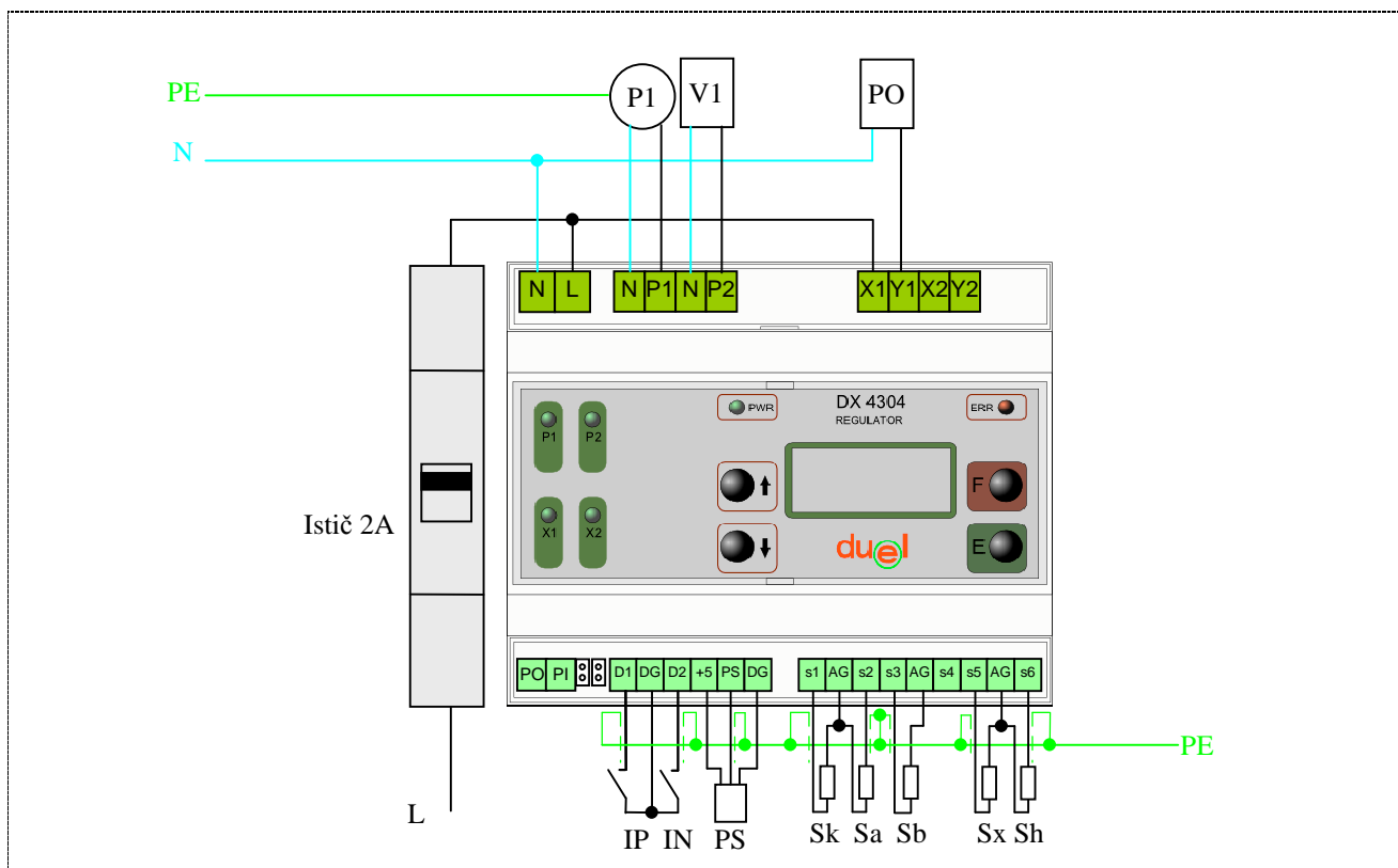
Obr.28 Príklad zapojenia regulátora DX4304 (svorkovnice sú pod krytom) pre sústavu s prepínacím ventilom: Sk - snímač teploty kolektora, Sa, Sb - snímače teplôt výmenníkov, Sx - snímač teploty spätného toku, Sh - snímač teploty pomocného ohrevu, PS - snímač tlaku, PO - stýkač, ktorý spína pomocný ohrev (napr. trojfázovú špirálu), P1 - čerpadlo, V1 - prepínací ventil, IP - impulzný prietokomer, IN - prepínanie leto/zima
