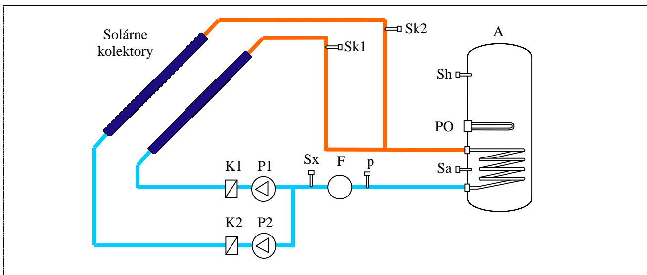
Obr.4 Bloková schéma regulovanej sústavy s dvoma kolektorovými poliami: A - výmenník, Sk1, Sk2, Sa, Sx, Sh - snímače teploty, p - snímač tlaku, F - snímač prietoku, PO - pomocný ohrev, P1,P2 - čerpadlá, K1,K2 - spätné klapky
