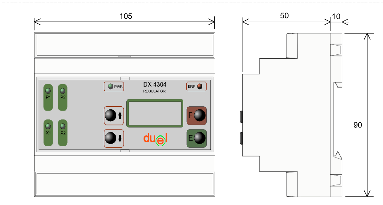
Obr.25 Rozmery prístroja DX4304
