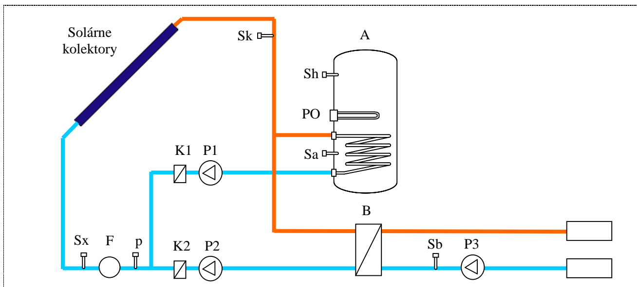
Obr.3 Bloková schéma regulovanej sústavy so samostatnými čerpadlami: A,B - výmenníky, Sk, Sa, Sb, Sx, Sh - snímače teploty, p - snímač tlaku, F - snímač prietoku, PO - pomocný ohrev, K1,K2 - spätné klapky, P1,P2,P3 - čerpadlá
