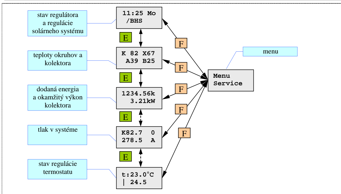
Obr.10 Prepínanie medzi zobrazovaniami stavu regulácie a menu
