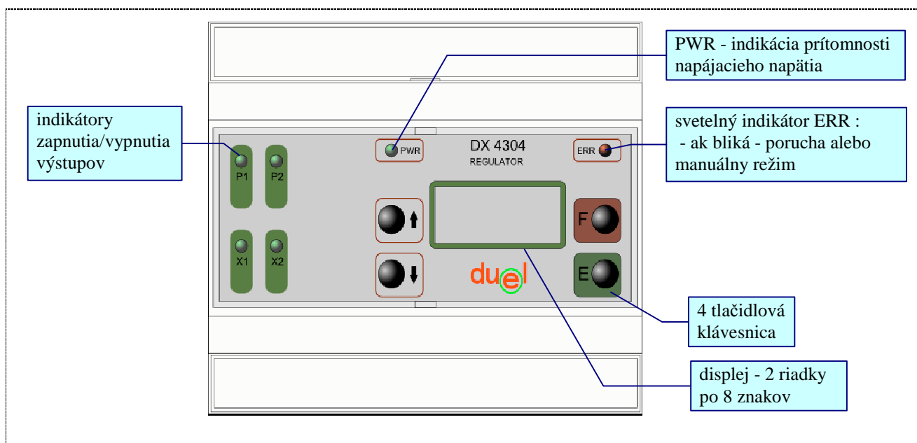
Obr.9 Predný panel regulátora DX4304
