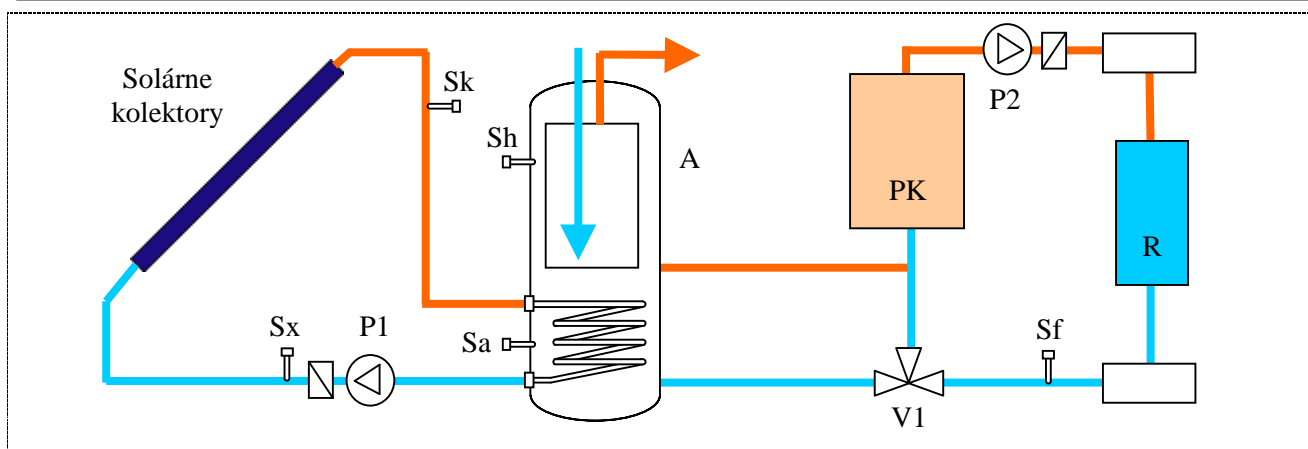
Obr.6 Príklad schémy regulovanej sústavy s diferenciálnym ohrevom: A - akumul. nádrž, PK - kotol, Sk, Sx, Sa, Sh, Sf - snímače teploty, V1 - prepínací ventil, P1, P2 - čerpadla, R - vykurovacie telesa
