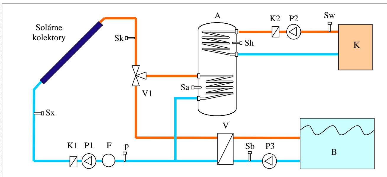
Obr.2 Bloková schéma regulovanej sústavy s prepínacím ventilom: A - výmenník (bojler), V - doskový výmenník (pre bazén B), Sk, Sa, Sb, Sh, Sx, Sw - snímače teploty, p - snímač tlaku, F - snímač prietoku, V1 - prepínací ventil, P1,P2,P3 - čerpadlá, K - kotol (alebo krb), K1,K2 - spätné klapky
