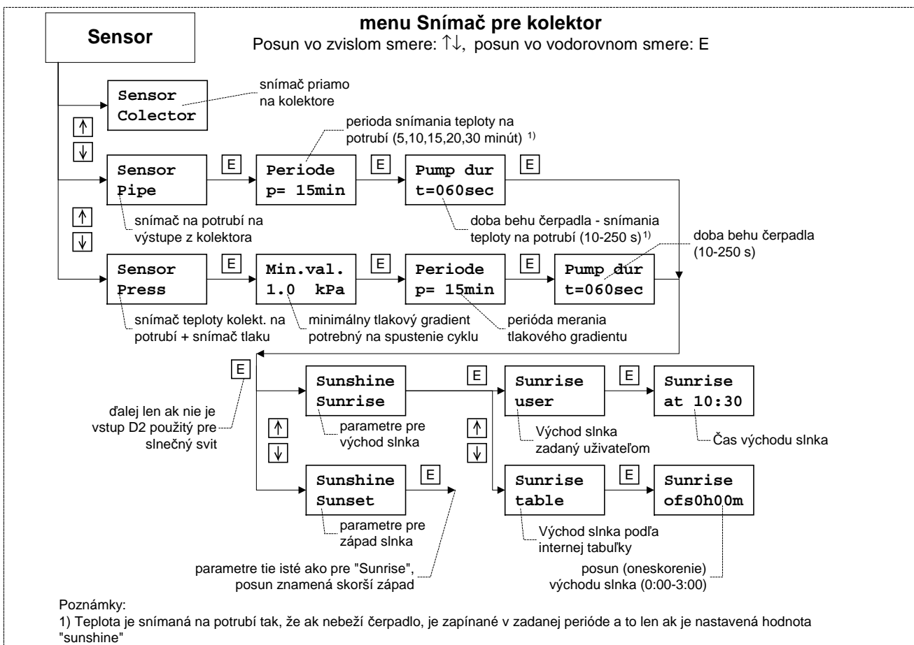
Obr.15 Menu "Sensor" - pre snímajúce teploty kolektora
