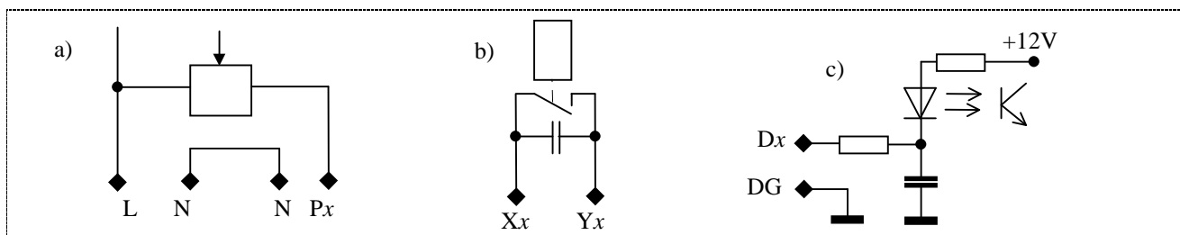
Obr.27 Zapojenia prístroja DX4304: a) výstupy P1-P2, b) výstupy X1-X2, c) digitálne vstupy D1 a D2
