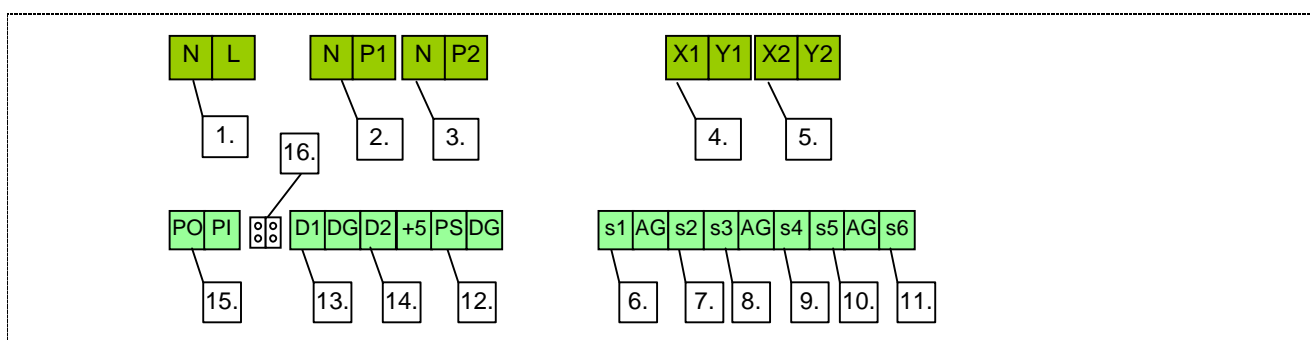
Obr.26 Zapojenie svorkovnice regulátora DX4304
