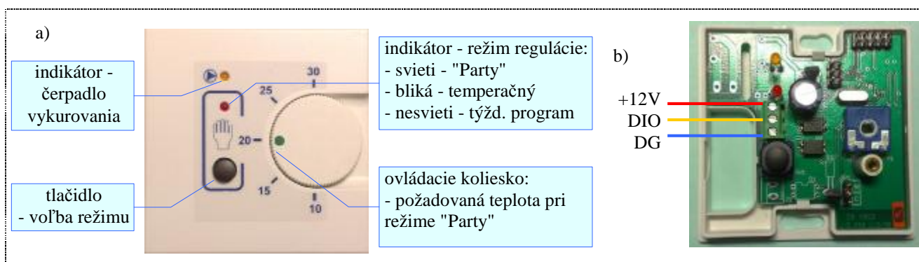
Obr.42 Priestorový snímač teploty DX1081: a) pohľad spredu, b) pohľad dovnútra a pripojenie k DX4232
