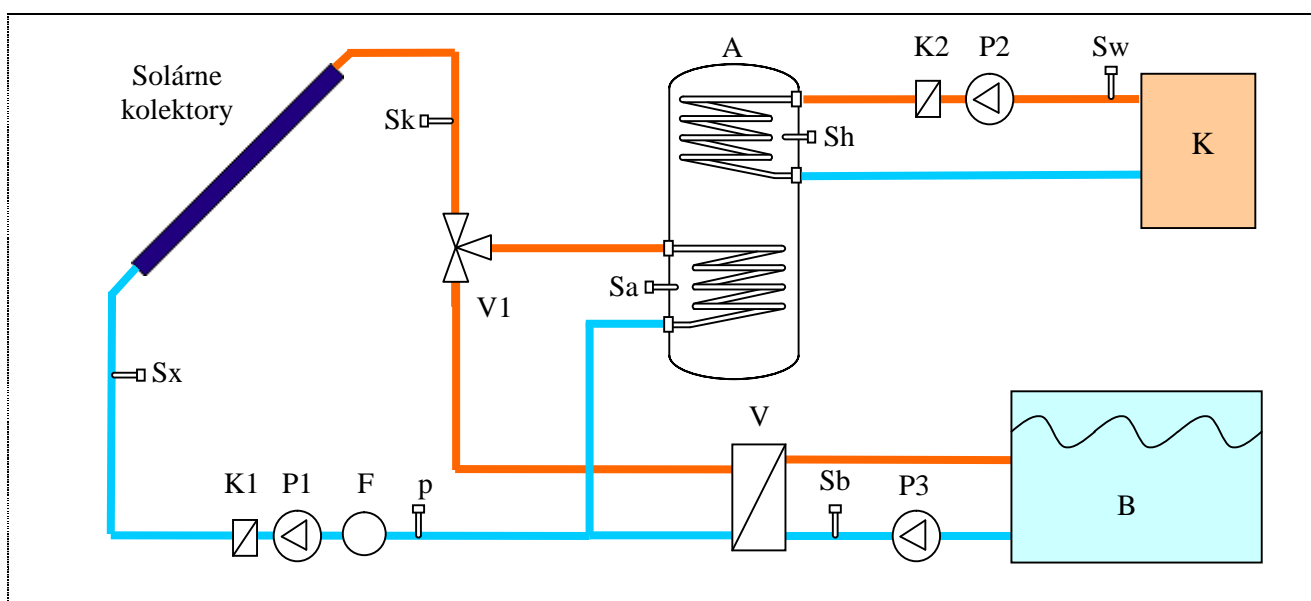
Obr.2 Hydraulická schéma regulovanej sústavy s prepínacím ventilom: A - výmenník (bojler), V - doskový výmenník (pre bazén B), Sk, Sa, Sb, Sx, Sh, Sw - snímače teploty, p - snímač tlaku, F - snímač prietoku, V1 - prepínací ventil, P1,P2,P3 - čerpadla, K - kotol (alebo krb), K1,K2 - spätné klapky
