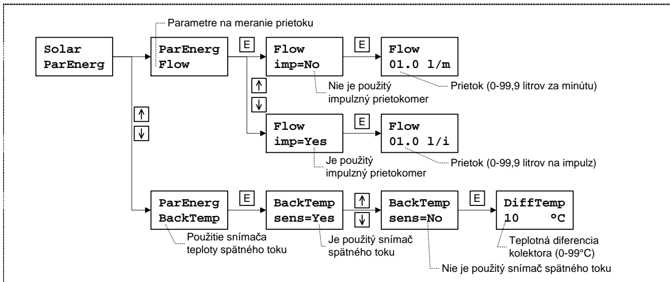
Obr.24 Menu "ParEnergy" - parametre pre meranie solárnej energie
