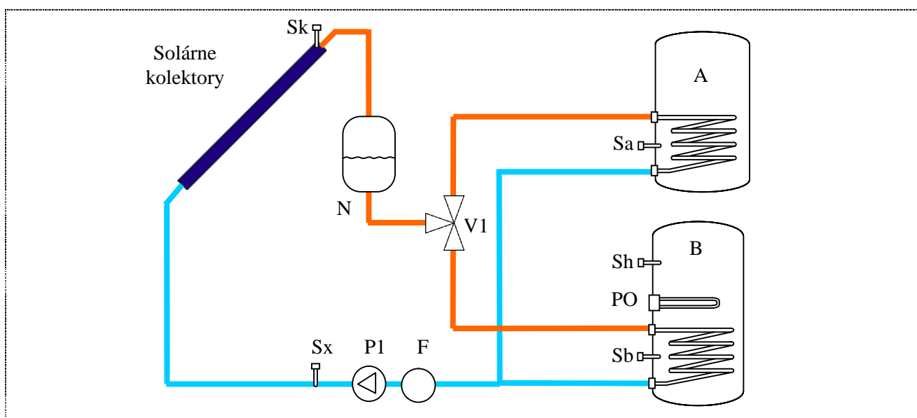
Obr.6 Hydraulická schéma regulovanej sústavy Drain-Back s pomocným ohrevom: N - nádrž pre kvapalinu kol. okruhu, A - akumul. nádrž, B - bojler, Sk, Sx, Sa, Sb, Sh - snímače teploty, F - snímač prietoku, PO - pomocný ohrev (napr. elektrická špirála), V1 - prepínací ventil, P1 - čerpadlo
