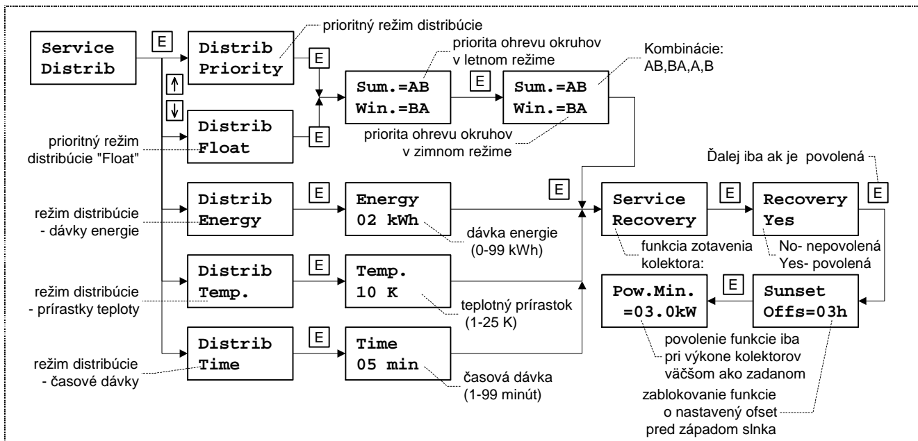
Obr.22 Menu "Distrib" - distribučné režimy
