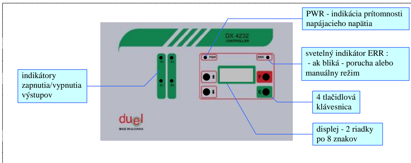
Obr.13 Predný panel regulátora DX4232
