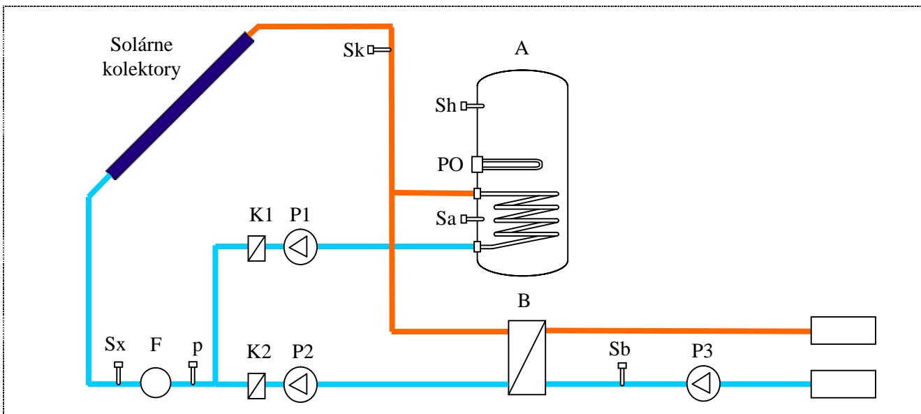
Obr.3 Hydraulická schéma regulovanej sústavy so samostatnými čerpadlami: A,B - výmenníky, Sk, Sa, Sb, Sx, Sh - snímače teploty, p - snímač tlaku, F - snímač prietoku, PO - pomocný ohrev, K1,K2 - spätné klapky, P1,P2,P3 - čerpadlá
