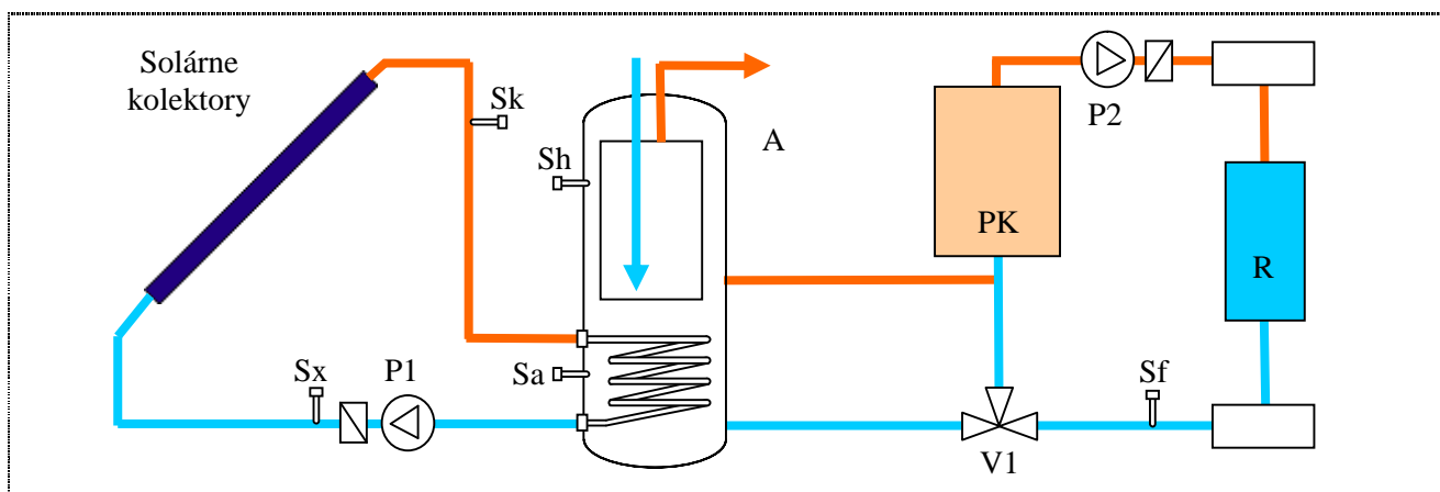
Obr.8 Príklad schémy regulovanej sústavy s diferenciálnym ohrevom: A - akumul. nádrž, PK - kotol, Sk, Sx, Sa, Sh, Sf - snímače teploty, V1 - prepínací ventil, P1, P2 - čerpadla, R - vykurovacie teleso
