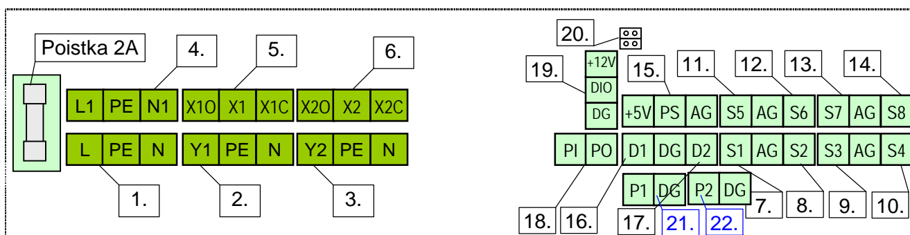
Obr.36 Zapojenie svorkovnice regulátora DX4232
