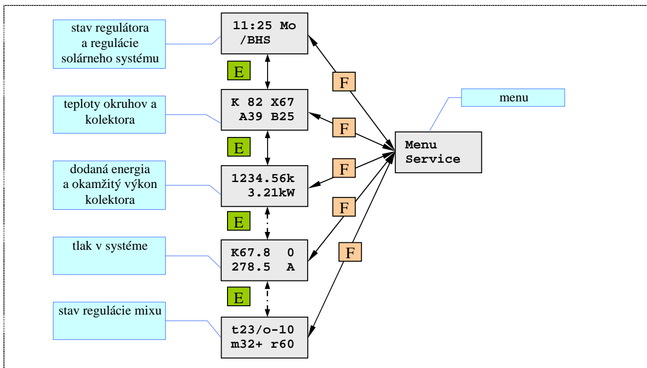
Obr.14 Prepínanie medzi zobrazovaniami stavu regulácie a menu
