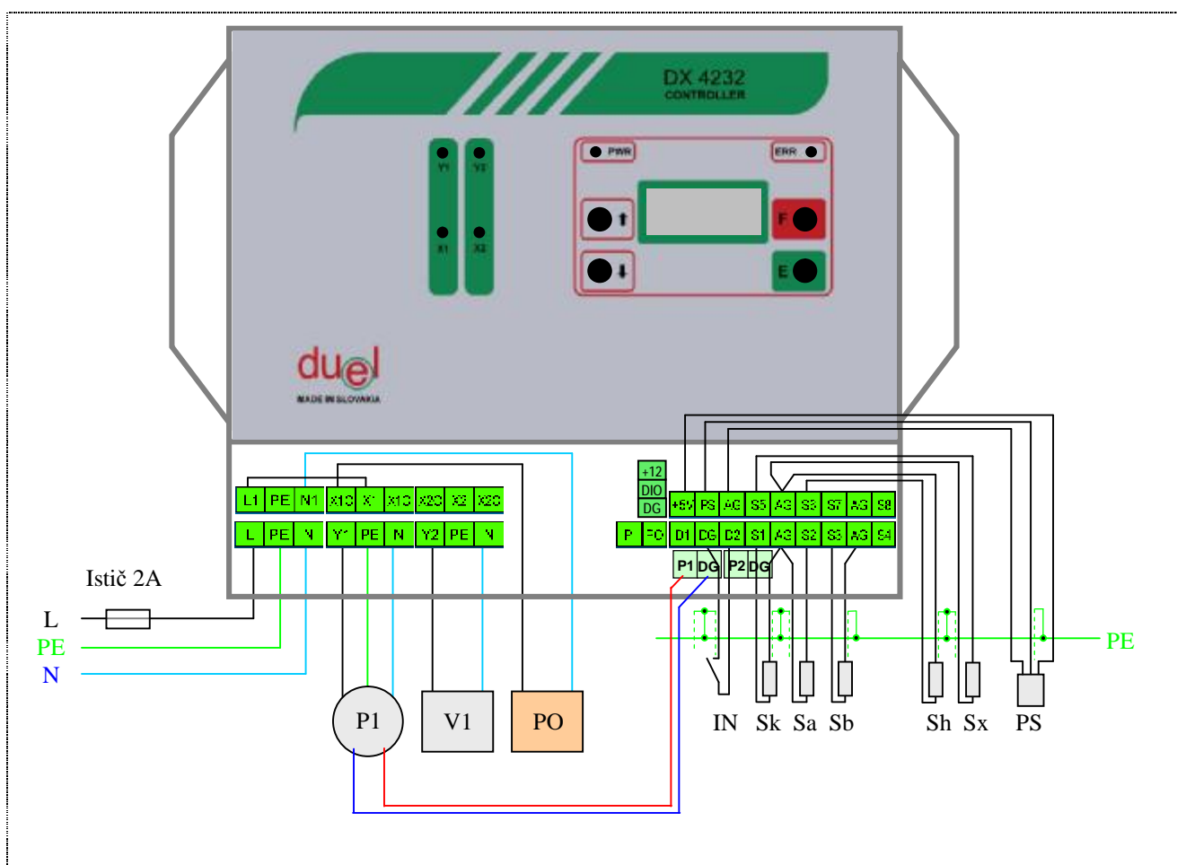
Obr.38 Príklad zapojenia regulátora DX4232 (svorkovnice sú pod krytom) pre sústavu s prepínacím ventilom: Sk - snímač teploty kolektora, Sa, Sb - snímače teplôt výmenníkov, Sx - snímač teploty spätného toku, Sh - snímač teploty pomocného ohrevu, PS - snímač tlaku, P1 - čerpadlo, V1 - prepínací ventil, IN - prepínanie leto/zima, PO - stýkač, ktorý spína pomocný ohrev
