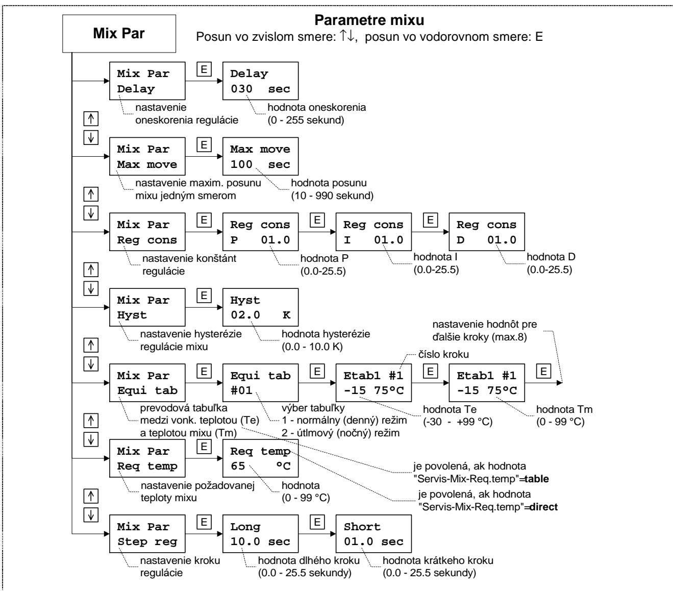
Obr.18 Menu "Mix Par" - parametre pre Mix
