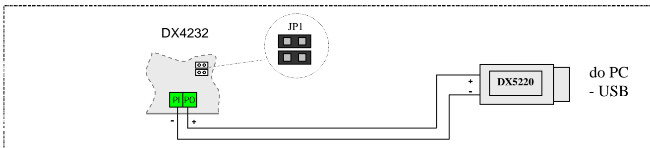
Obr.39 Pripojenie prístroja k PC s vnútorným napájaním (na PI-PO je naprázdno približne 14V, po pripojení prevodníka je na PI-PO 2,7V).
