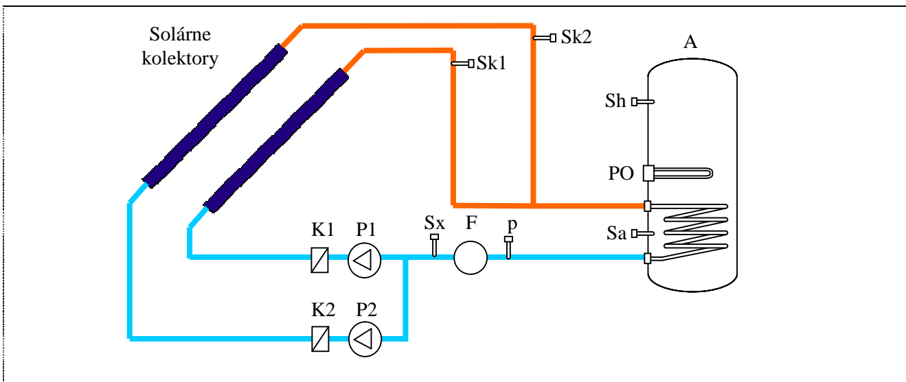
Obr.4 Hydraulická schéma regulovanej sústavy s dvoma kolektorovými poliami: A - výmenník (boljer), Sk1, Sk2, Sa, Sx, Sh - snímače teploty, p - snímač tlaku, F - snímač prietoku, PO - pomocný ohrev, P1,P2 - čerpadlá, K1,K2 - spätné klapky
