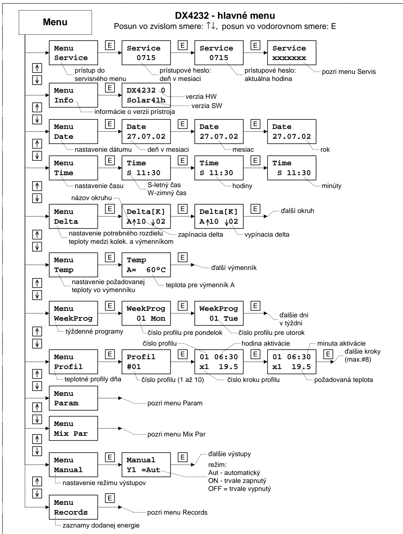
Obr.16 Menu regulátora DX4232 - menu pre servis je popísané na Obr.19
