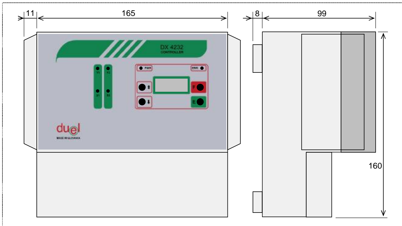
Obr.35 Rozmery prístroja DX4232
