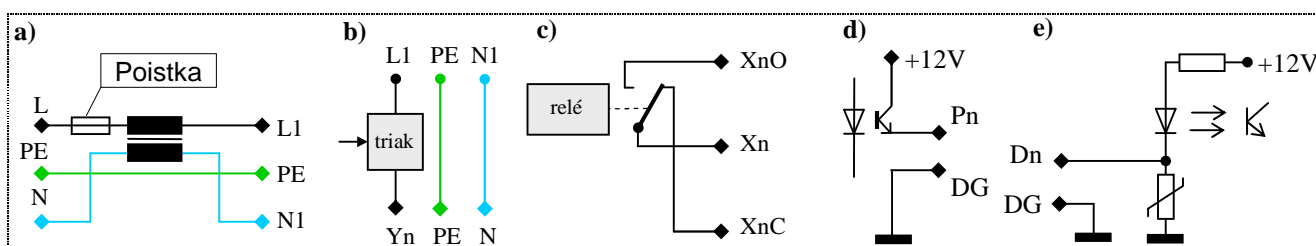
Obr.37 Zapojenia prístroja DX4232: a) prepojenie vstupného napätia b) výstupy Y1-Y2, c) výstupy X1-X2, d) PWM riadiace signály P1-P2, e) digitálne vstupy D1 a D2
