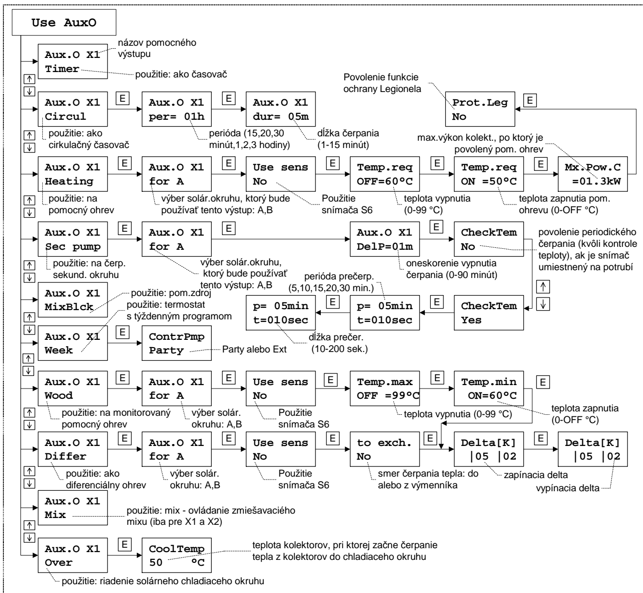
Obr.23 Menu "Use AuxO" - konfigurácia a parametre pomocných výstupov
