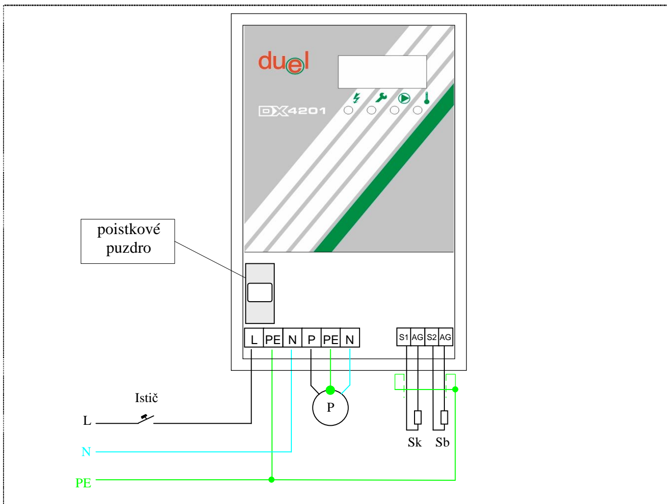
Obr.14 Príklad zapojenia regulátora DX4201 (svorkovnica a poistkové puzdro sú pod krytom): Sk - snímač teploty kolektora, Sb - snímač teploty výmenníka, P - čerpadlo
