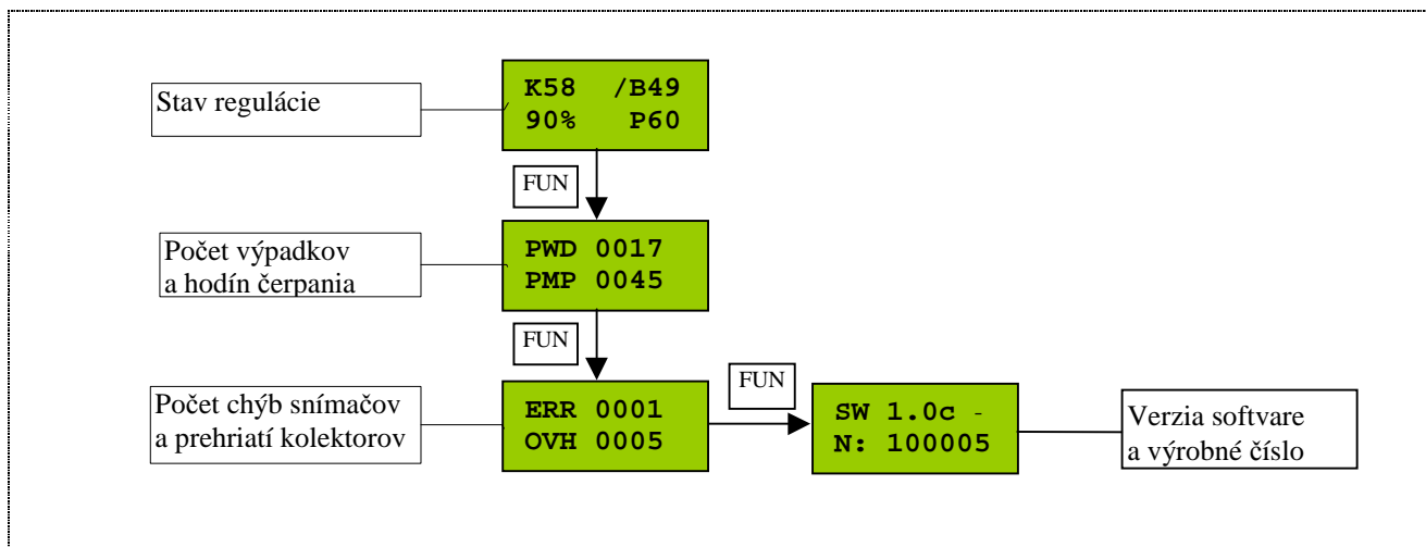
Obr.7 Prepínanie medzi zobrazovaním stavu regulácie a štatistických údajov
