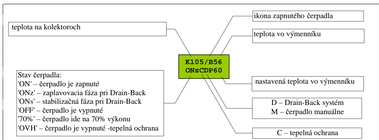
Obr.8 Zobrazenie stavu regulácie
