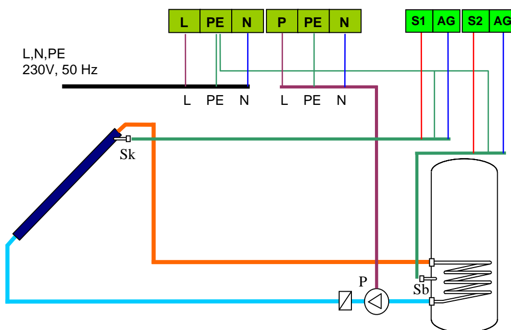
Obr.12 Doporučené zapojenie regulátora DX4201
