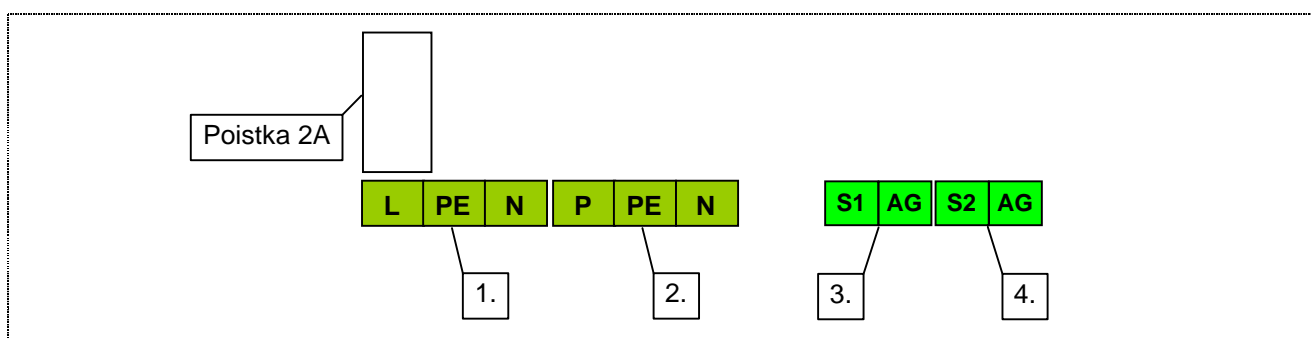
Obr.10 Zapojenie svorkovnice regulátora DX4201
