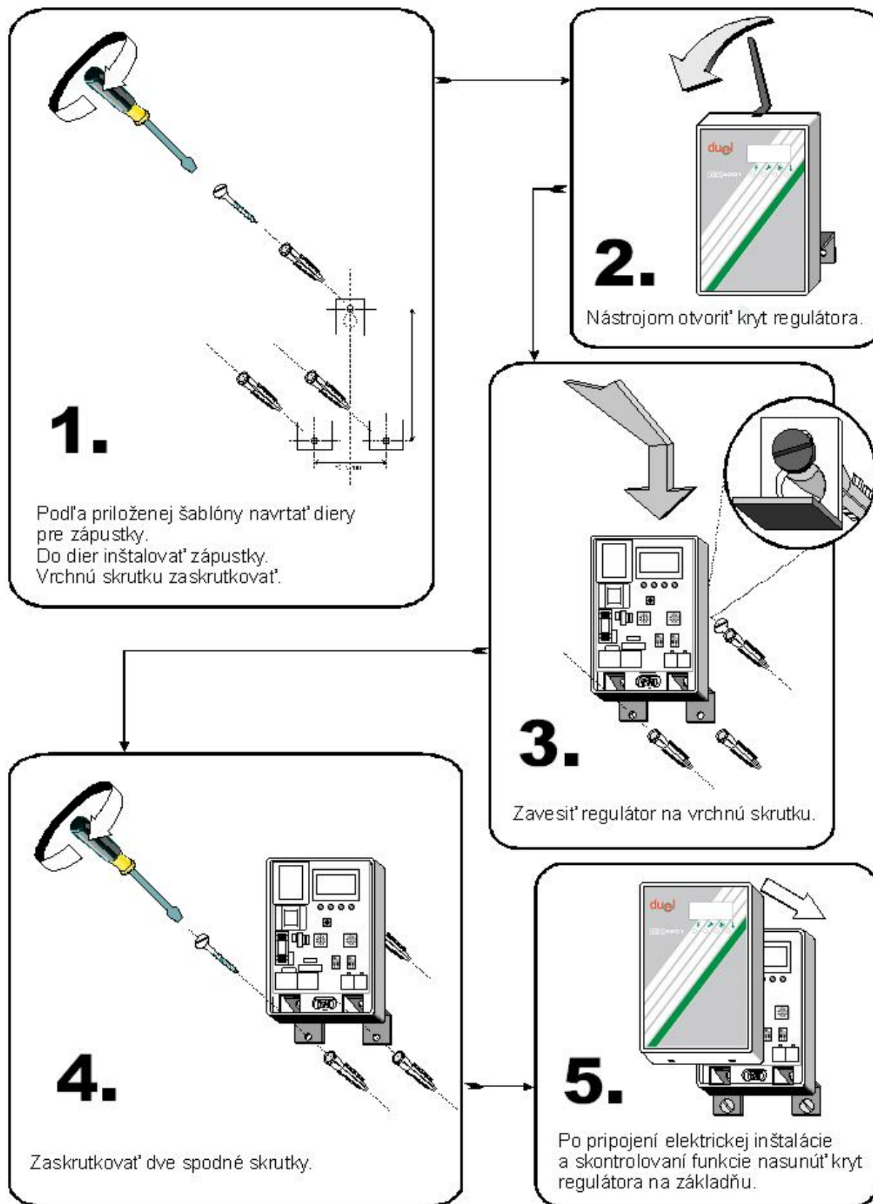
Obr.13 Montáž prístroja
