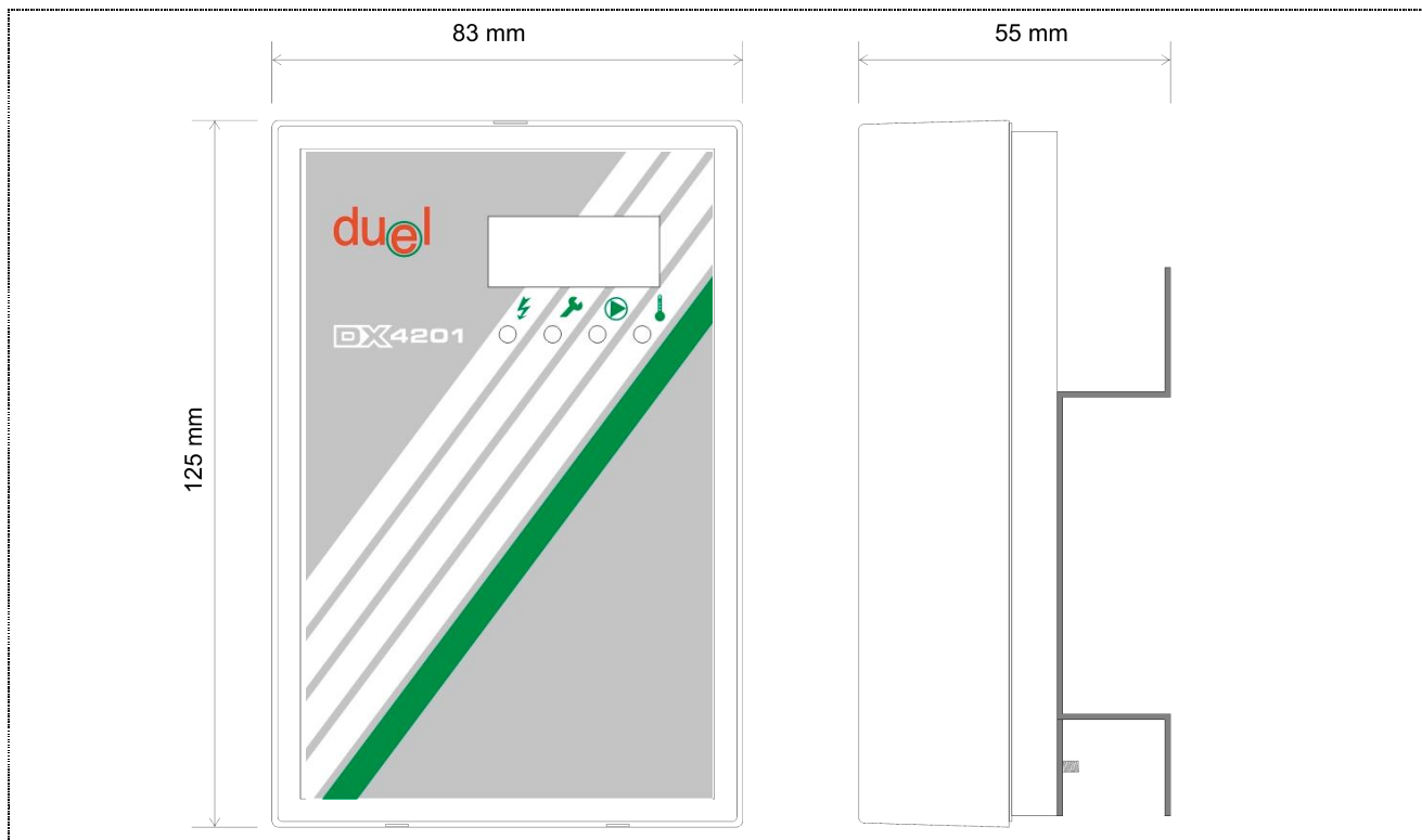
Obr.9 Rozmery prístroja DX4201
