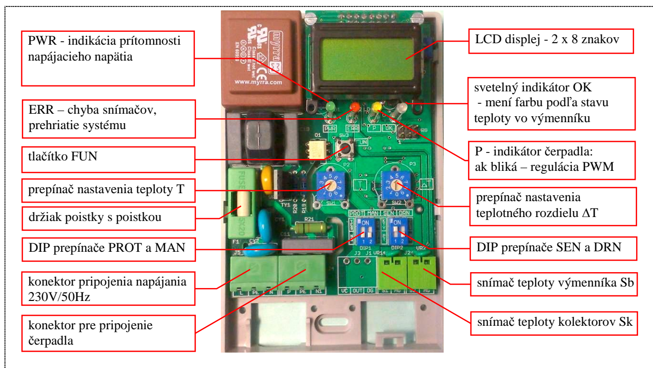
Obr.6 Nastavovacie a indikačné prvky regulátora DX4201
