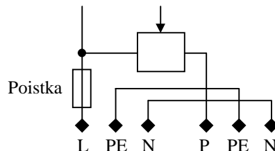
Obr.11 Zapojenie výstupu regulátora DX4201
