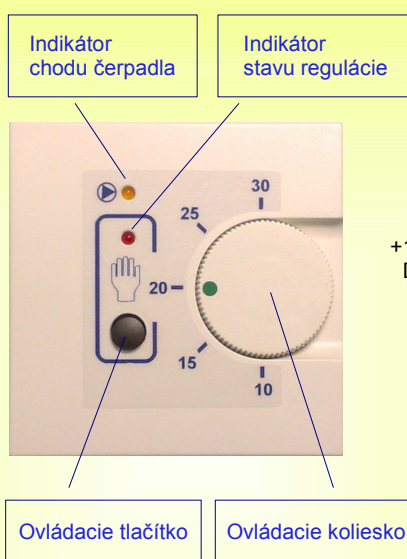
a) pohľad spredu a popis prvkov
